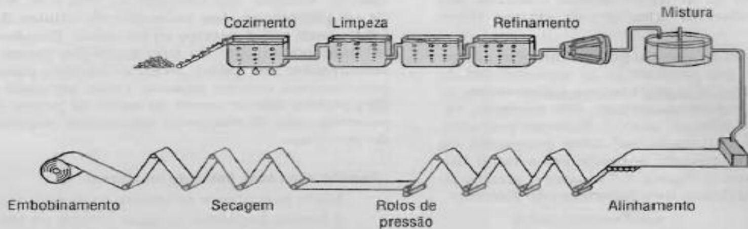
Figura 7.6 Seqüência de processos na manufatura de papel. Cada processo será arranjado fisicamente com a mesma seqüência.
